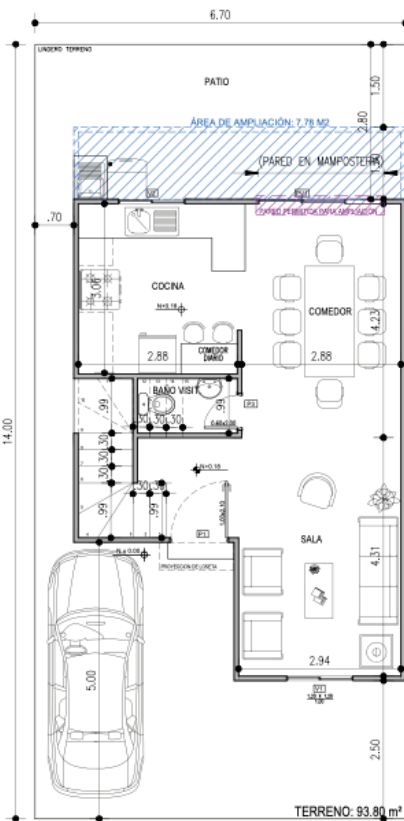
PLANTA BAJA AREA: 44.95 m²
